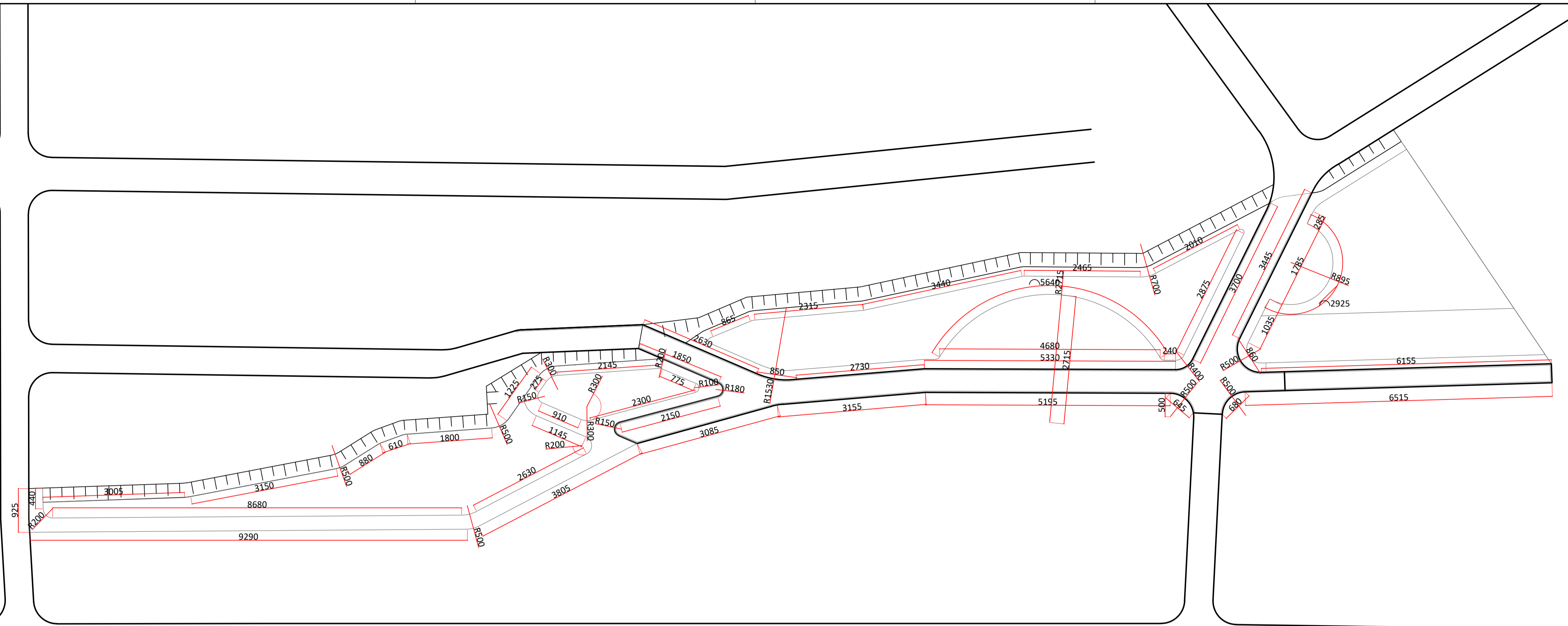
09 PLANTA BAIXA 1 : 500
