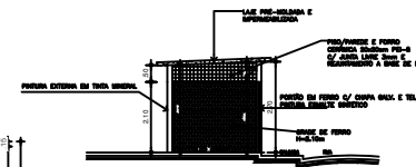
CORTE LM ABRIGO DE LIXO ESQ. 1:75
