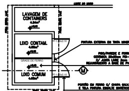
PLANTA BAIXA ABRIGO DE LIXO A=14,84m² ESQ. 1:75
