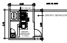
PLANTA BAIXA A=9,24m² ESQ. 1:75
