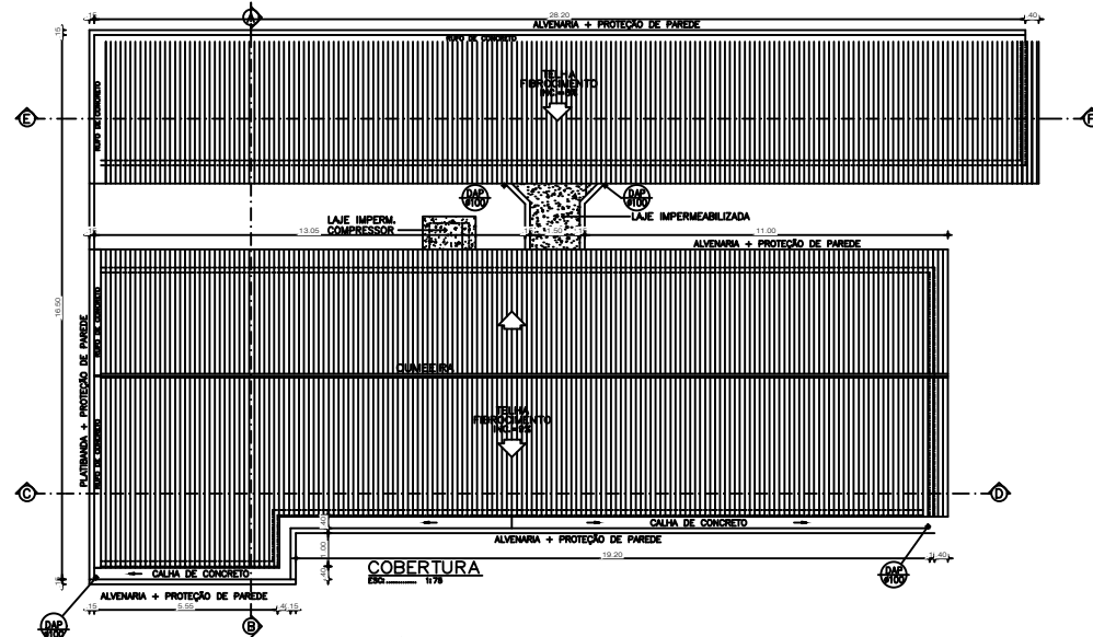
COBERTURA ABRIGO DE LIXO ESQ. 1:75
