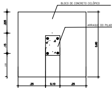
DETALHE DA FUNDAÇÃO)
