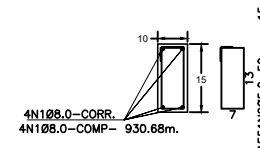
DETALHE DA CINTA C1(10x15) (159.20m) 5/ESCALA
