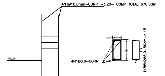
DETALHE DO PILAR) 5/ESCALA
