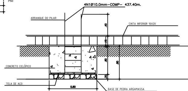
DETALHE DA FUNDAÇÃO) 5/ESCALA
