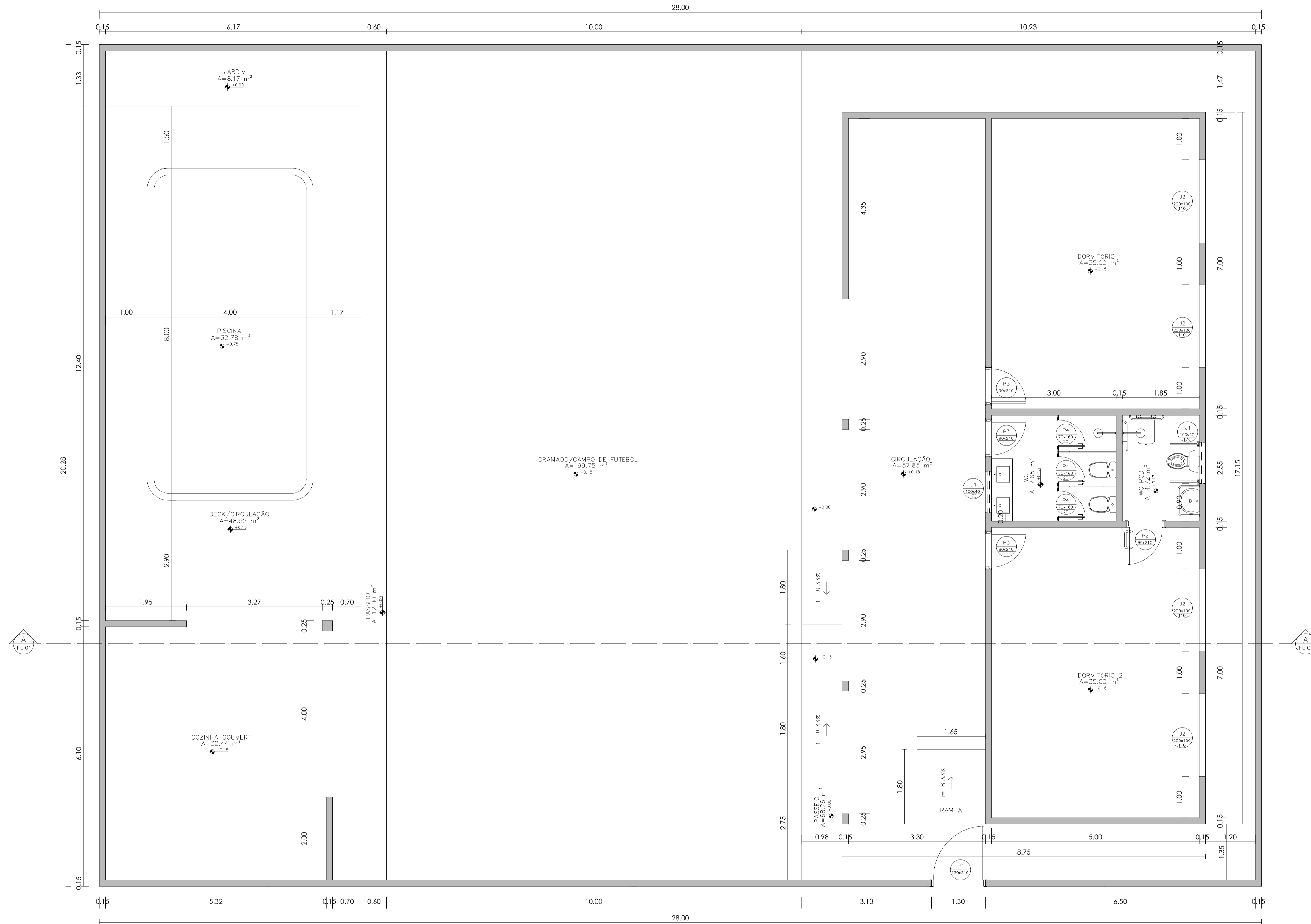
PLANTA BAIXA ESCALA - 1/50
