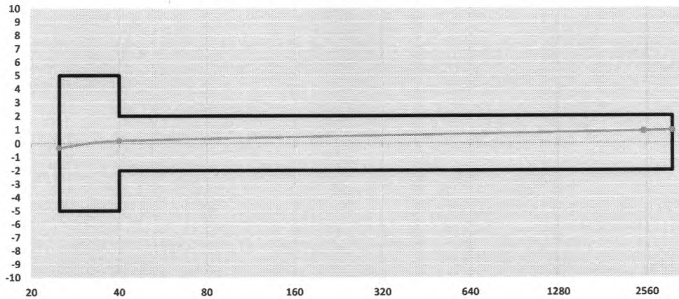
Curva de Erro - Laquam Q 3 =2,5 R100 H
