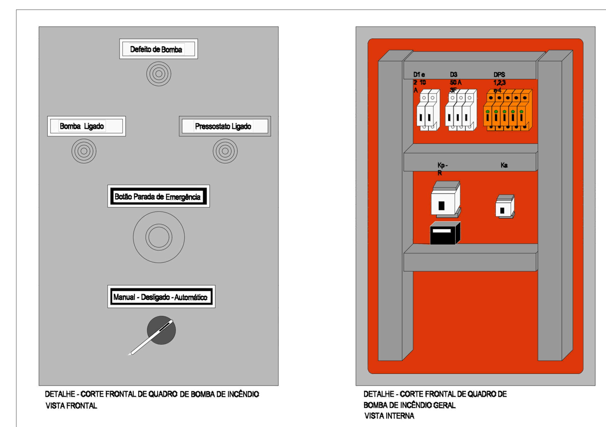
DETALHE DO PAINEL
