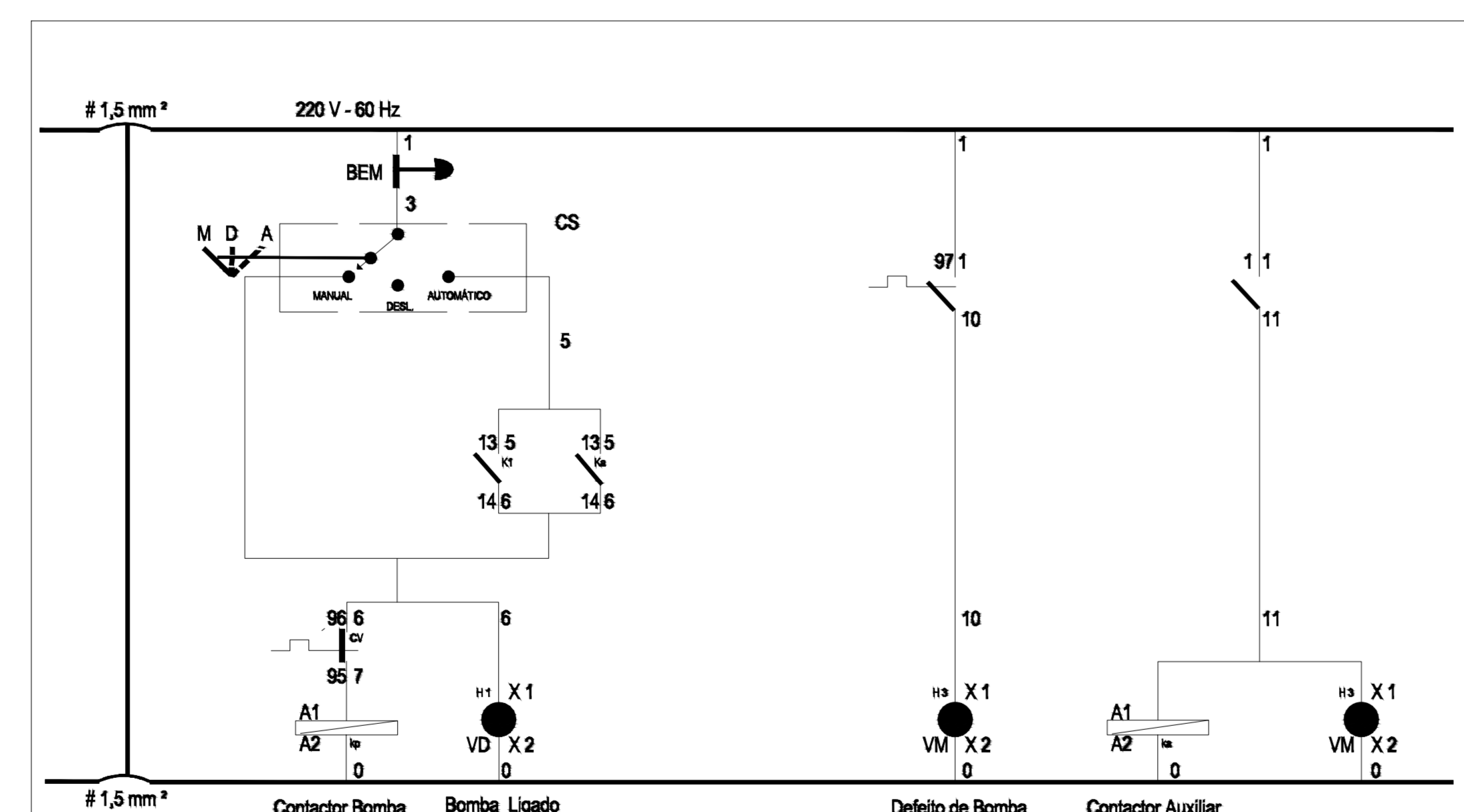
DETALHE DO DIAGRAMA UNIFILAR
