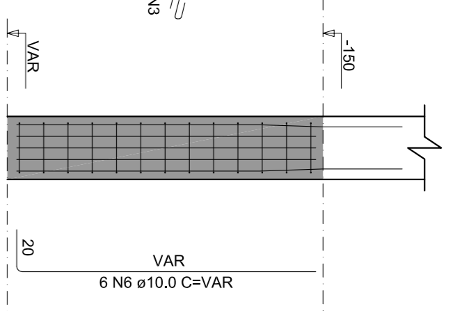
VISTA H ESC: 1/25
