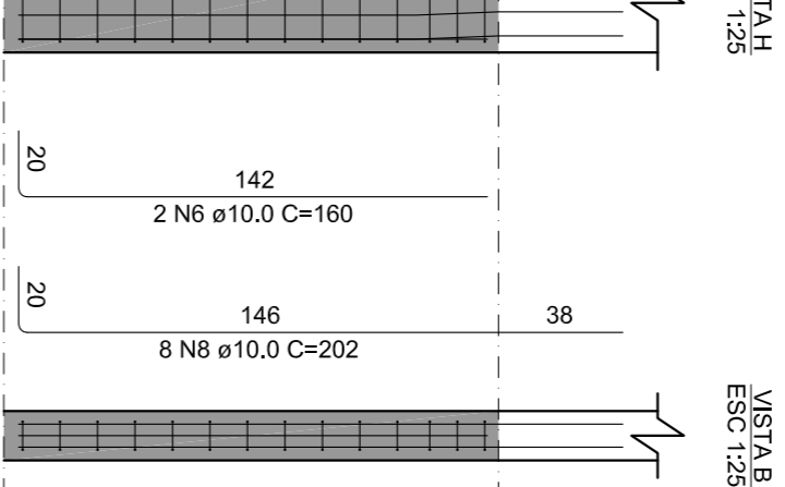
VISTA B ESC: 1/25
