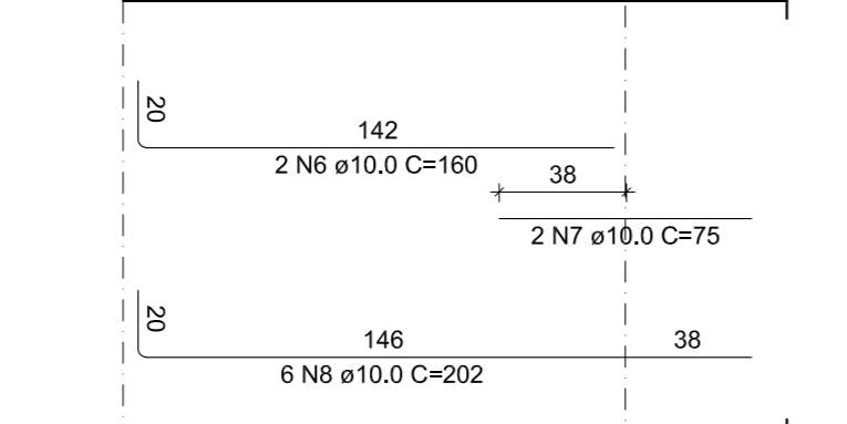
VISTA B ESC: 1/25
